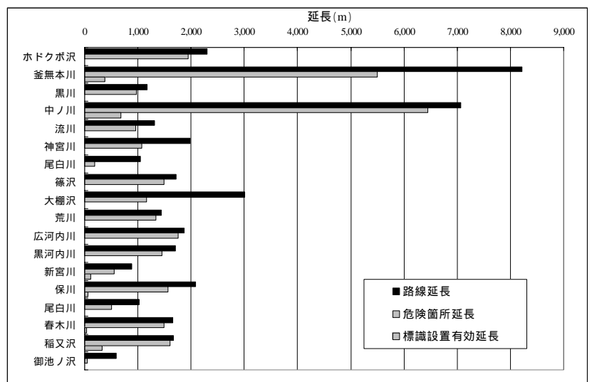
図3 工事用道路の延長と危険箇所の関係
