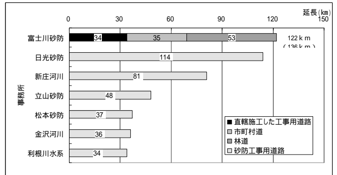
図1 砂防工用道路の直轄事務所別の延長比較
