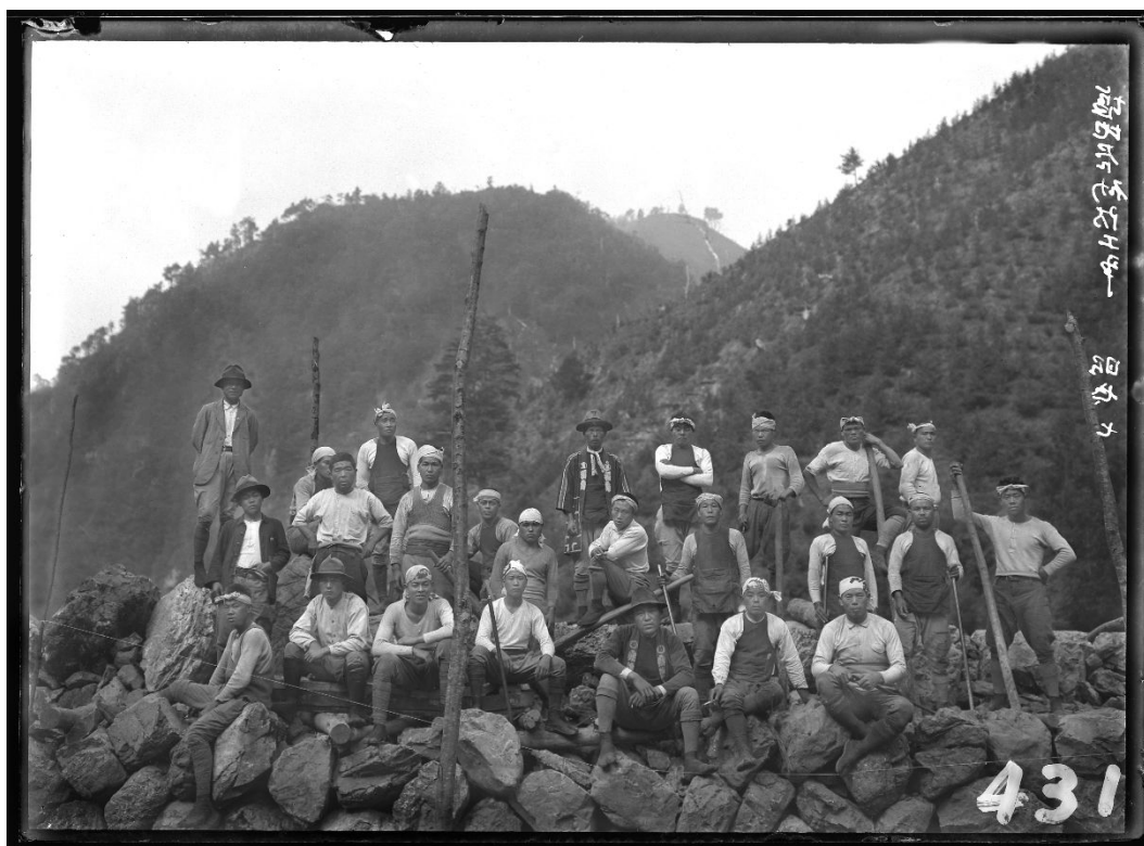
R219 シオジ谷 砂防工事(昭和7年7月)
