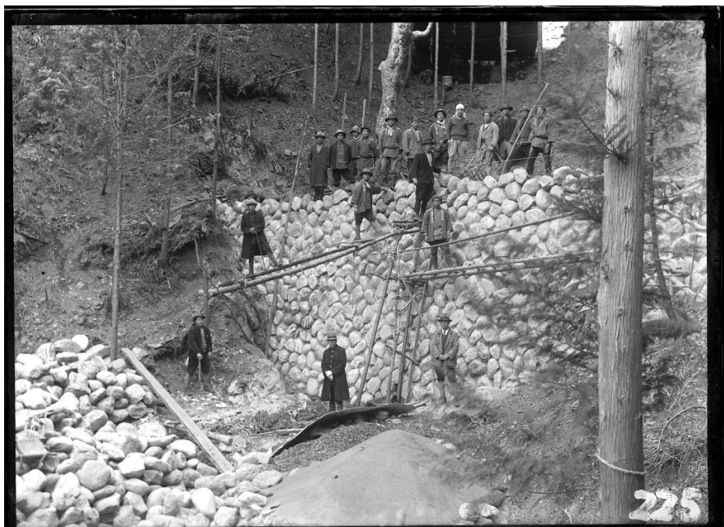
R251 水源林 石堰堤(施工中)(撮影時期不明)
