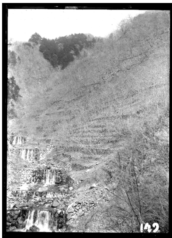
R272 場所不明 石堰堤(撮影時期不明)
