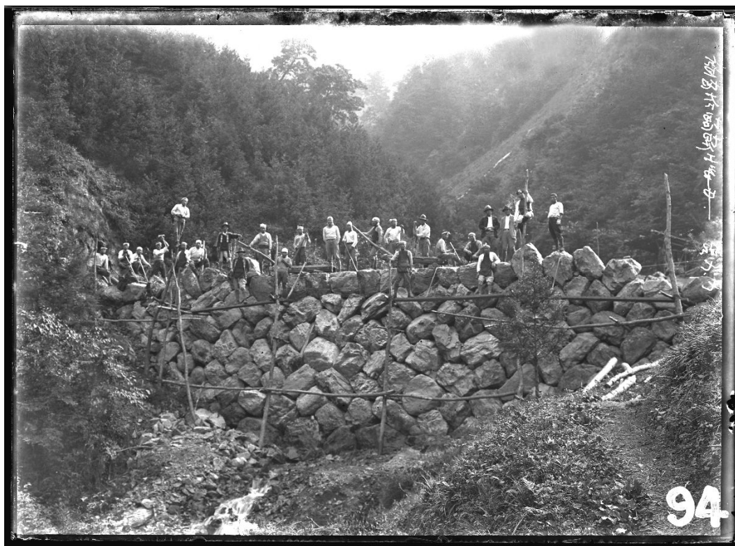
R218 シオジ谷 石堰堤(施工中)(昭和7年7月)
