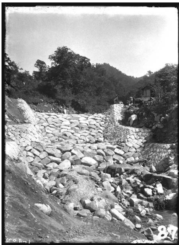
R258 柳沢 石堰堤(大正2年9月) 【諸戸北郎博士収集写真集 1026と同一写真】
