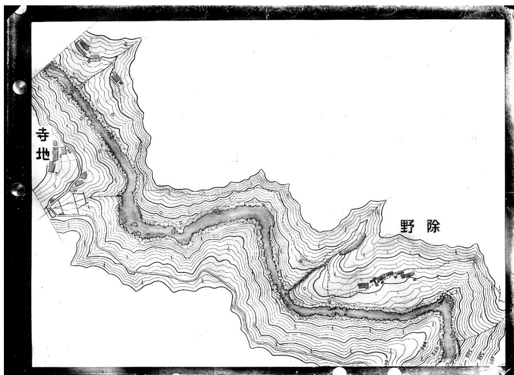
R228 寺地 地形図(撮影時期不明)
