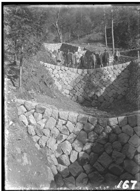
R208 サイグチ 石堰堤(昭和 7 年 11 月)
