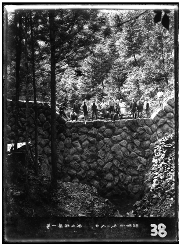
R202 ミズクボ沢 混合積石堰堤(昭和4年9月18日)
