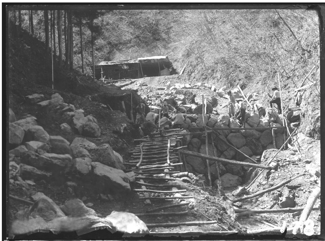
R212 手沢 石堰堤 臨時工事(昭和 10 年)
