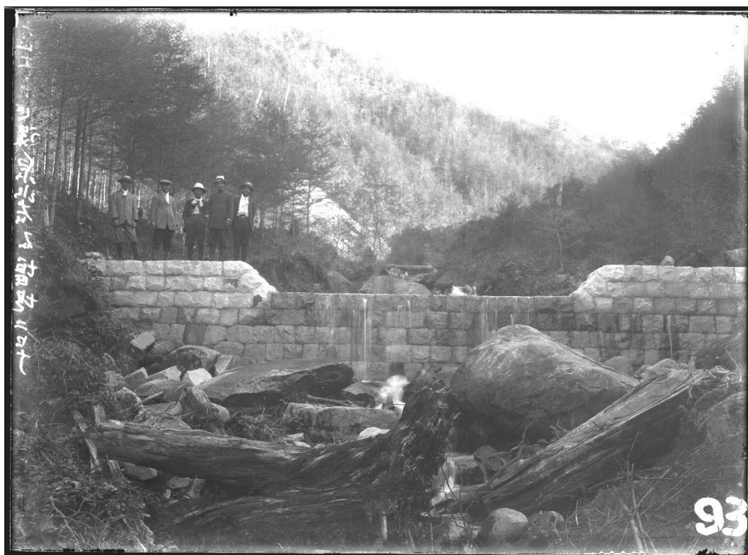
R155 センスイ谷 石堰堤 2号(大正 11 年 11 月)
