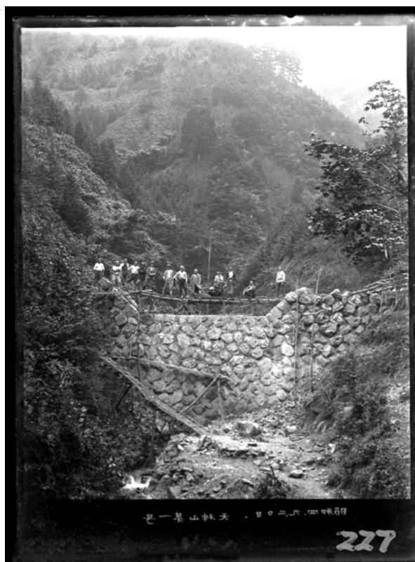
R196 天神山 1号堰堤(昭和4年9月20日)
