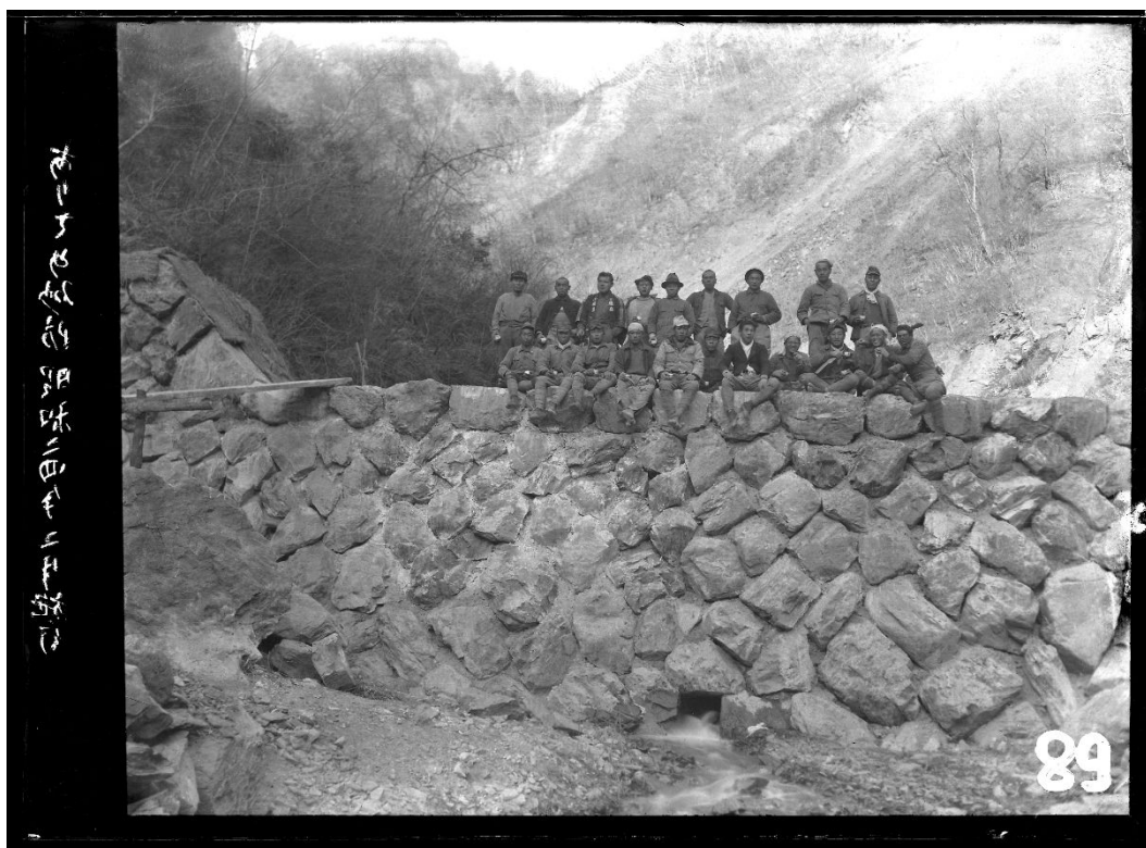
R184 ありさめ 練積堰堤 昭和 24 年 2 月施工(撮影時期不明)
