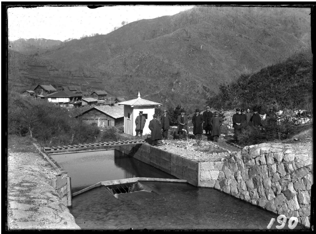
R082 カネバ沢 量水堰堤 府会議員一行(大正 5 年 11 月 20 日)
