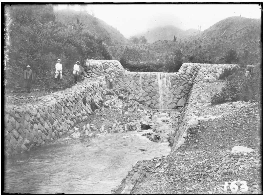
R079 カネバ沢 石堰堤(大正 4 年) 【諸戸北郎博士収集写真集 990 と同一写真】
