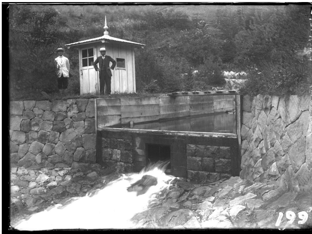
R075 カネバ沢 量水堰堤 (撮影時期不明)
