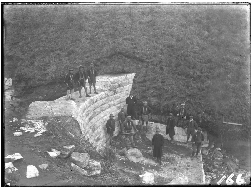
R068 シシネド沢 石堰堤(大正 5 年 12 年)
