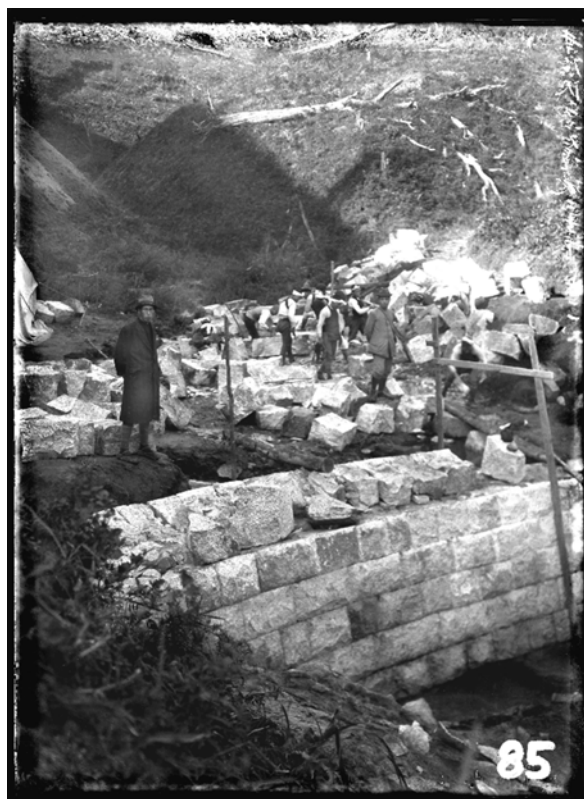
R057 ハビロ沢 石堰堤(施工中)(大正 5 年 11 月)
