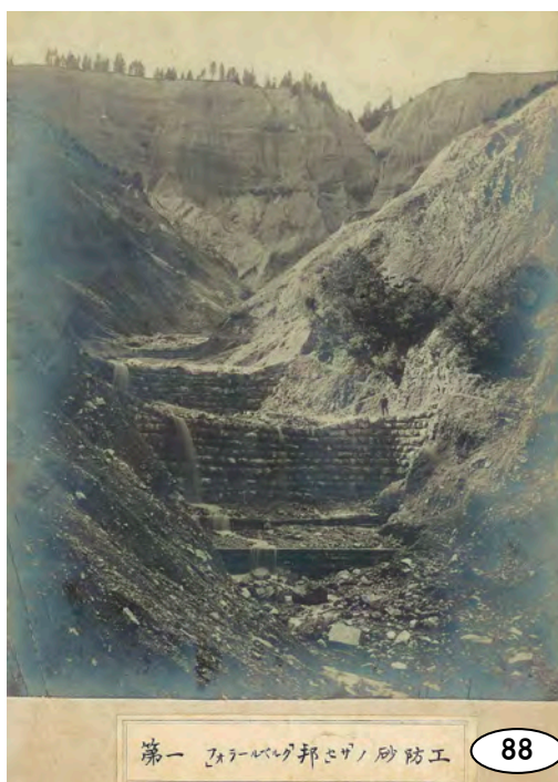
Verbauung der Schesa 「フォアールベルグ」邦「セサ」ノ砂防工
