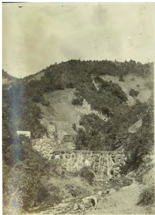
明神峠事業正峯坂澤 第一、三、五号堰堤並山腹石積工 大正十五年春施行 大正十五年秋堰
