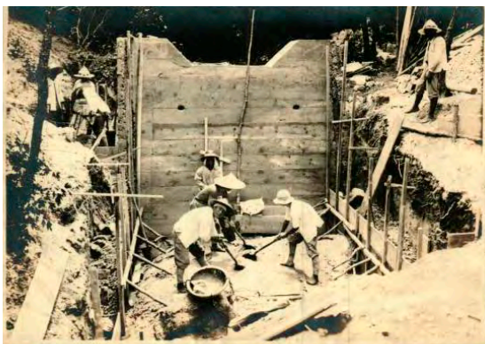
白坂Ⅱ-124, 混凝土土堰堤 側壁/練込
